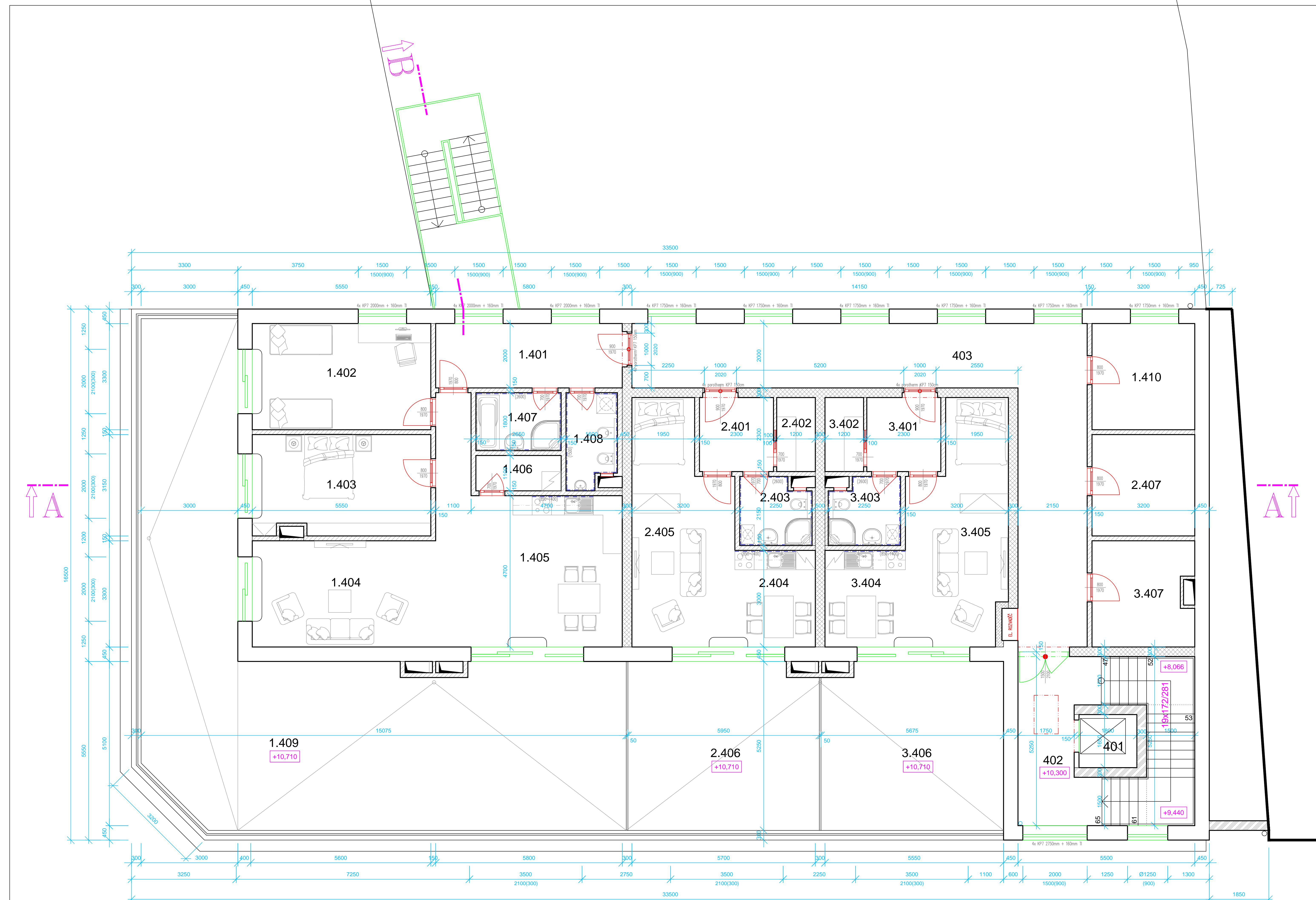
PŮDORYS 4.NP
